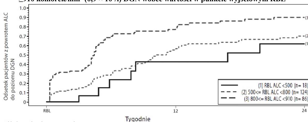
Ryc. 1 Metoda Kaplana-Meiera; odsetek pacjentów, u których nastąpił powrót do wartości \geq 910 komórek/ mm^3 ( 0,9 \times 10^9/l ) DGN wobec wartości w punkcie wyjściowym RBL
